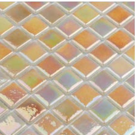
2008 250 ₺ +kdv 25 x 25 mm Plaka ebat : 31,5 x 31,5 cm Kutu : 1m 2 - 10 Plaka
